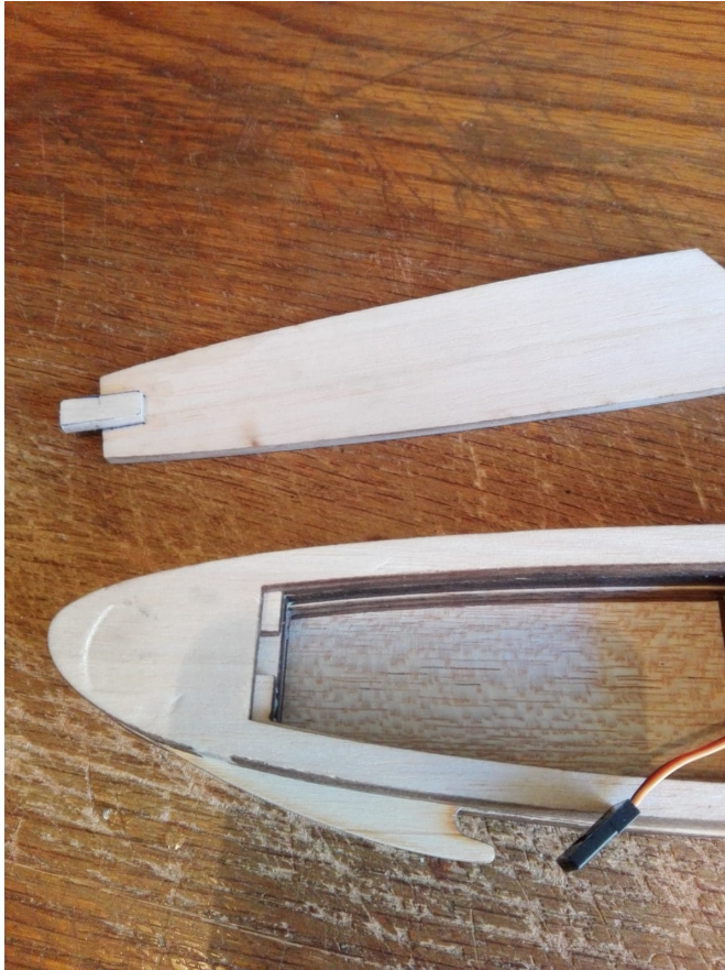
Bild 05: Abdeckung der RC-Anlage z.B. mit Magnetverschluss und Hochstarthaken
