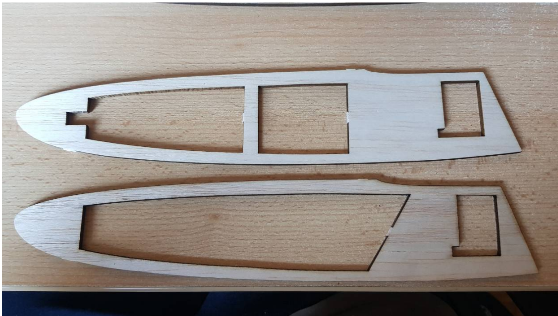
Bild 01: Rumpfaufbau großflächige Seitenteile. Man erkennt schon die späteren Servo-Sitze
